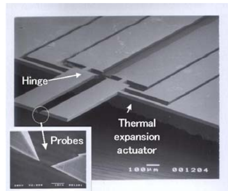
Nano-gripper
